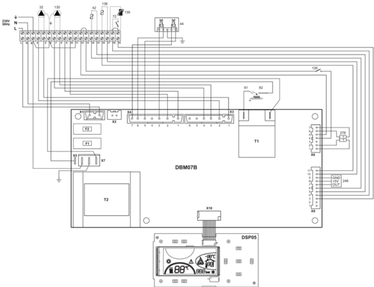
рис. 27 - Электрическая схема В
