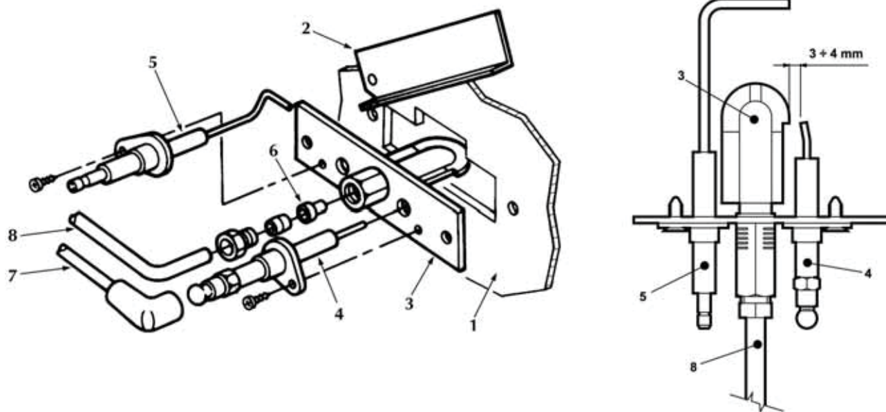
рис. 23 - Пилотная горелка
